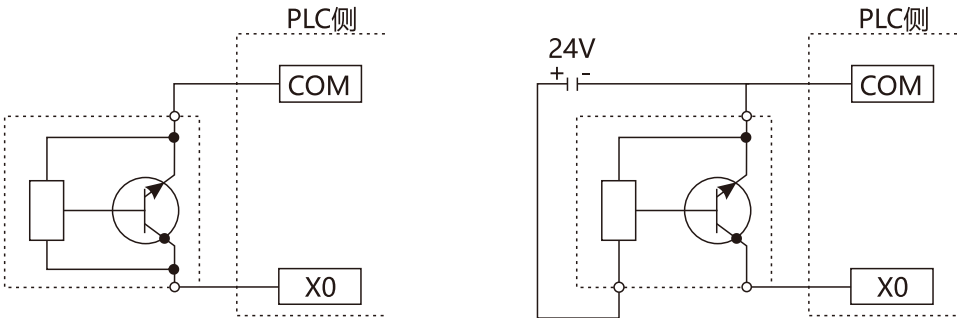
两线制（NPN型）接近开关接线图示例
