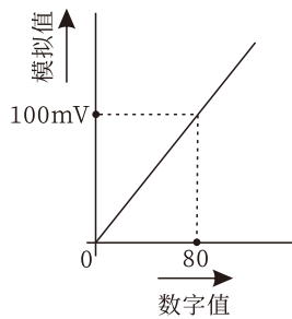
电压输出特性(0到5V)
