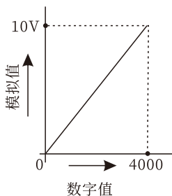
电压输出特性(0到10V)
