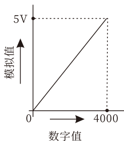
电压输出特性(0到5V)
