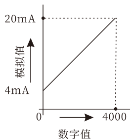
电流输出特性(4到20mA)
